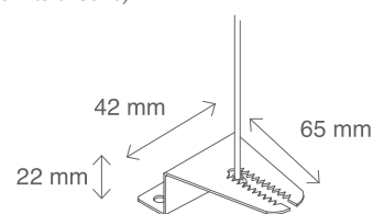
SQUADRETTA A Z CON MORSETTO (a richiesta)
