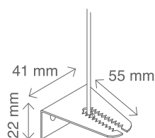
SQUADRETTA DI FISSAGGIO A PARETE CON MORSETTO (a richiesta)
