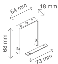
CAVALLOTTO A SOFFITTO (fornito di serie)
