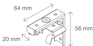
SUPPORTO A SCOMPARSA A SOFFITTO (a richiesta)
