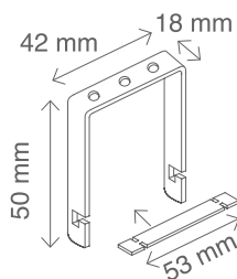
CAVALLOTTO SUPPORTO A SOFFITTO (fornito di serie)
