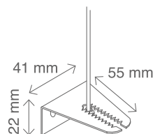
SQUADRETTA DI FISSAGGIO A PARETE CON MORSETTO (a richiesta)
