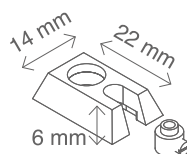
SQUADRETTA IN POLICARBONATO CON TENDICAVO
