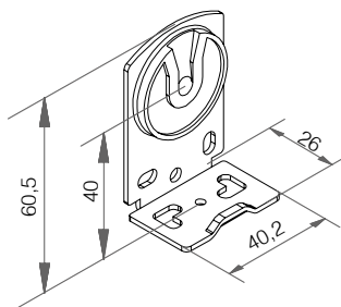
STAFFA LATO RISCONTRO
