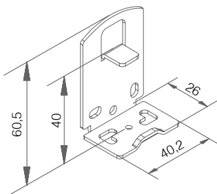
STAFFA LATO COMANDO
